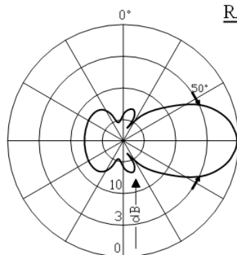
E-PLANE
