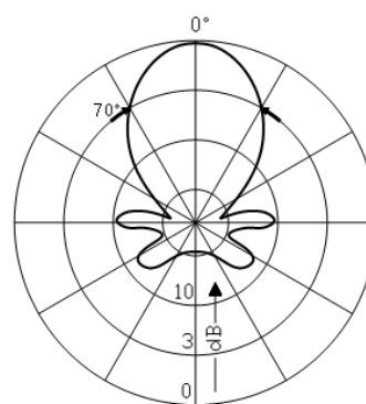
H-PLANE
