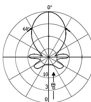
H-PLANE
