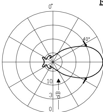
E-PLANE
