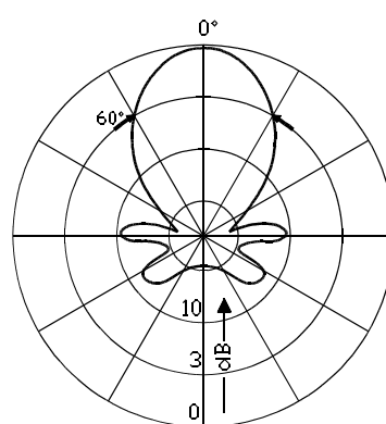
H-PLANE
