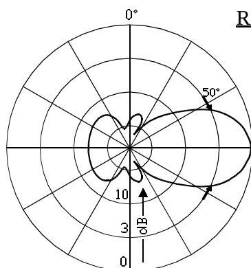
E-PLANE
