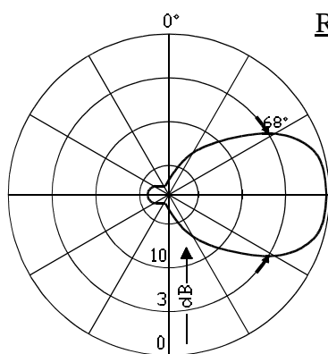
E-PLANE
