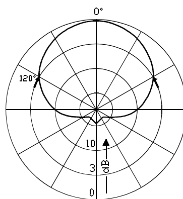
H-PLANE
