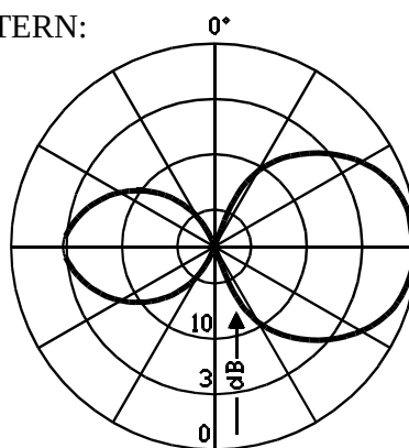
H-PLANE
