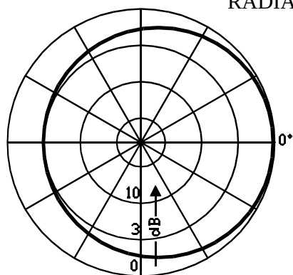
E-PLANE
